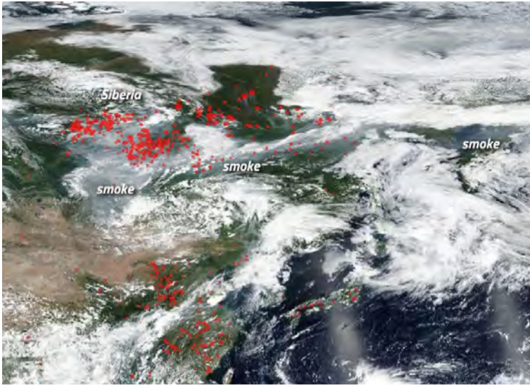
Útbreiðsla skógarelda í Síberíu og reyks af þeirra völdum. /Mynd NOAA/NASA.
