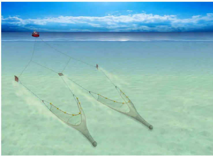
Mynd 3. Togari að draga tvö troll.
