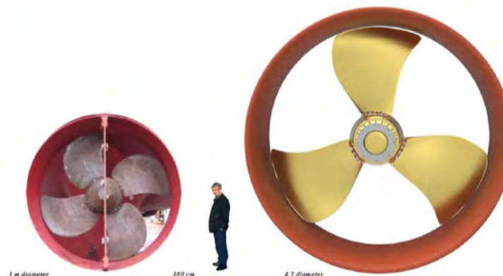
Mynd 2. Hér sjáum við 3ja metra skrúfu sem var undir gamla Páli Pálssyni (smíðuðum í Japan 1972) og 4,7 metra skrúfu undir nýja Páli Pálssyni, smíðuðum í Kína 2018. Mædurinn á myndinni er 1,8 metrar.
