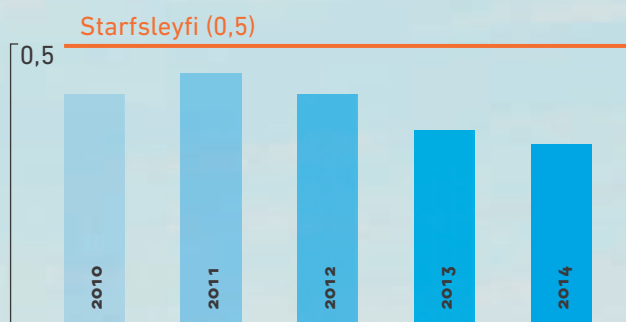
Losun flúors (kg / mt Al)
