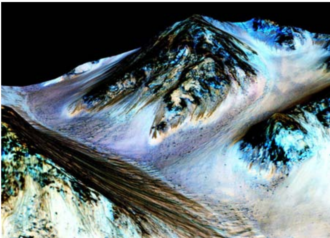
Grenjandi hlíðar Mars. Rákirnar myndast út frá árstíðabundnu flæði vatns á yfirborðinu. MYND/NASA/JPL
