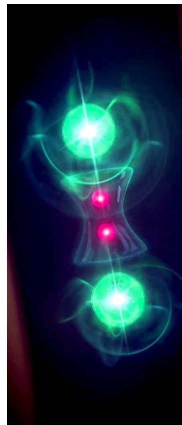
Draugaleg virkni virðist vera staðreynd en brýtur þó ekki gegn afstæðiskenningu Einsteins, enda ómögulegt að senda upplýsingar í gegnum skammtaflækju.
