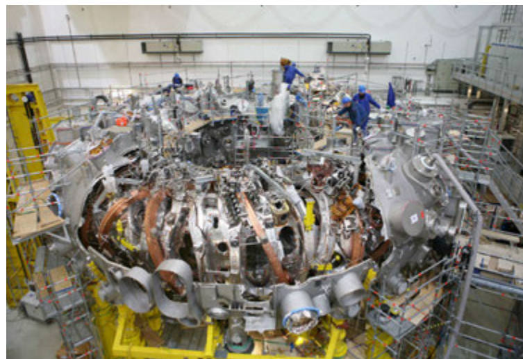
Hin hræðilega fallega Stellarator-vél. Frasin „fegurðin kemur innan frá“ hefur aldrei átt jafn vel við.
