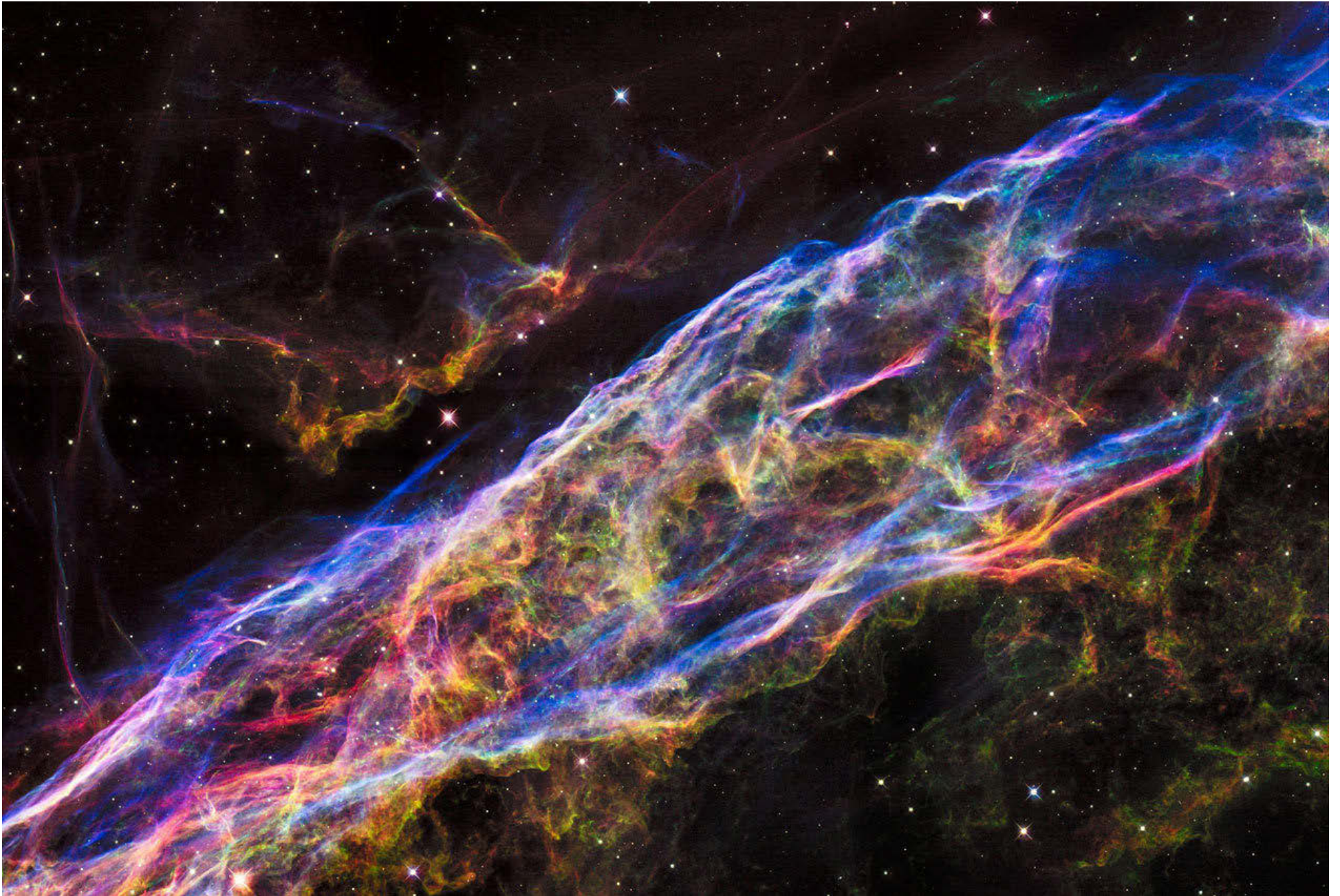
Blæjan Fyrir um 8.000 árum sprakk stjarna í 2.100 ljósára fjarlægð í stjörnumerkinu Svaninum. Leifar hennar dreifðust um geiminn og rækust síðan á efni milli stjarnanna á 1,5 milljóna km hraða á klukkustund og tóku þá að glóa. Litadýrðin í þessum gasþráðum stafar af mismunandi og misheitu efni. MYND: NASA/ESA OG HUBBLE HERITAGE TEAM
