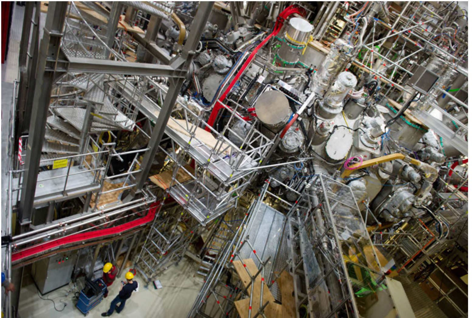
Hin ófrýnilega Wendelstein 7-X var ræst í fyrsta skipti á dögunum og það með sögulegum árangri. MYND/EPA
