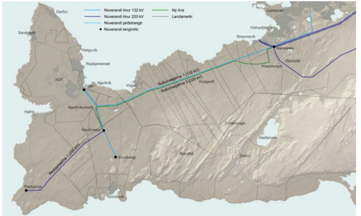
Linur Landsnets á Reykjanesi núverandi sem nýjar, núverandi línur má betur sjá á heimasíðu LN á forsiðu „Heildarflutningur núna“. MYND/VERKFRÆÐISTOFAN EFLA
